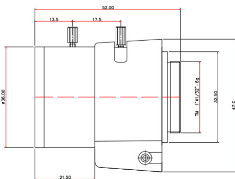
镜头尺寸平面图:
